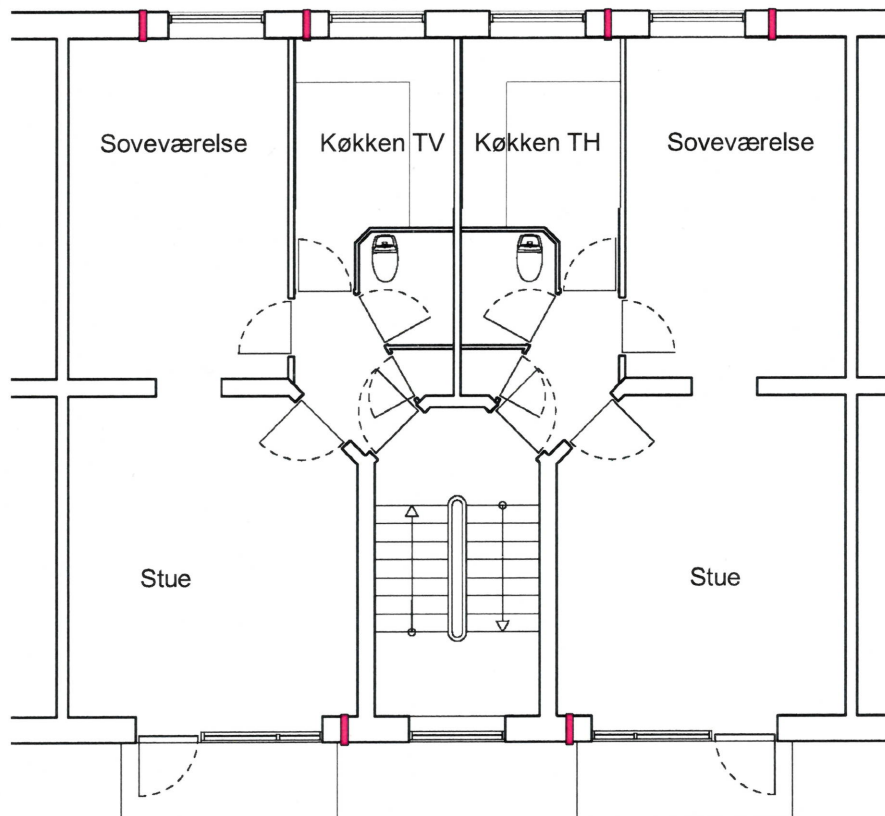
Plan Lejlighed til venstre og til højre 1:100
