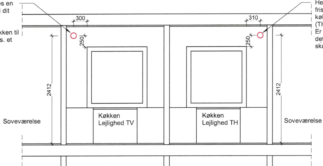
Snit Køkken 1:50
